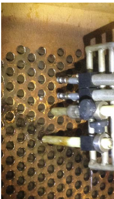
Tvätt av stora värmväxlare i samarbete med Vattenfall. Operatören fäster munstycket från roboten i hålen som ska tvättas. Därefter sker tvätt med iller som matas ut automatiskt i jämn hastighet. Operatören slipper bli nersmutsad av tvättvatten och tvättresultatet blir jämnare och bättre.
